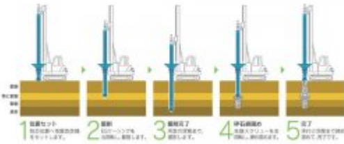
エコジオ工法 施工順序
